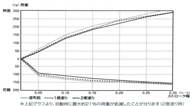
ダンパーテスターによる試験 ドライループforダンパー塗布前、塗布後のデータ比較
